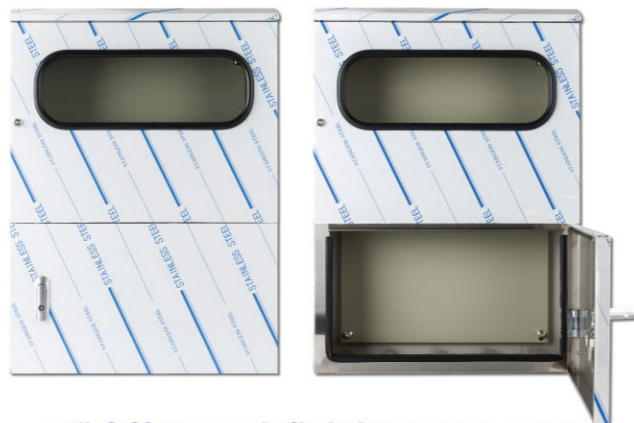
스텐 옥외 SCT 3상 계량기(STS 201, 1.2T)
